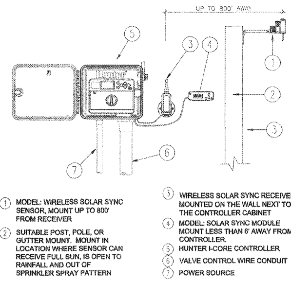
12 WIRELESS SOLR SYNC N.T.S.
